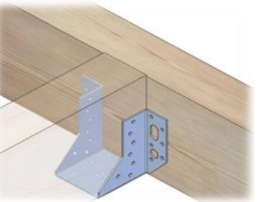
Supporte Para Vigas mod.363
